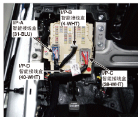
54.仪表板左侧
