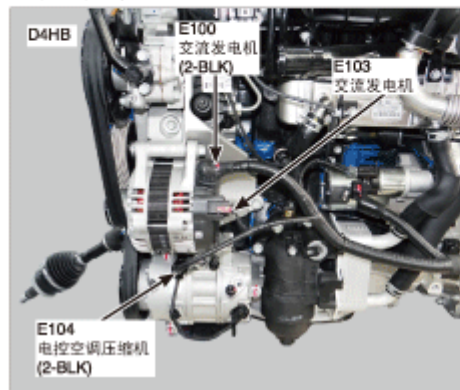
49.发动机左侧
