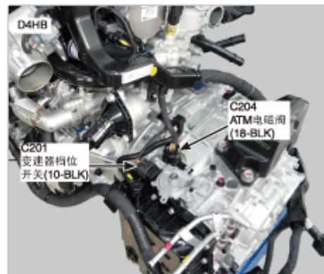
51.变速器顶部
