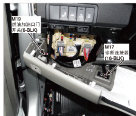
53.仪表板左侧
