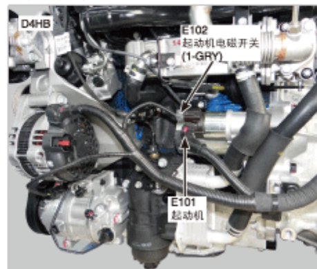
50.发动机左侧
